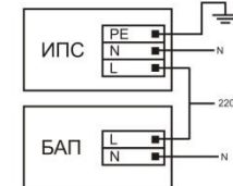
Рис.2 (с блоком аварийного питания)
