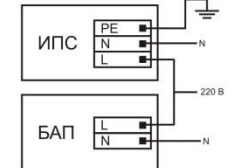
Рис.2 (с блоком аварийного питания)
